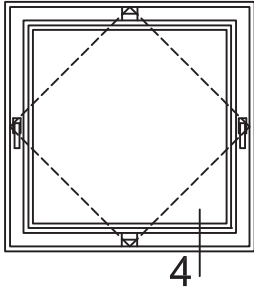
Pivot Window System Detail Pivot Pencere Sistem Detayı
