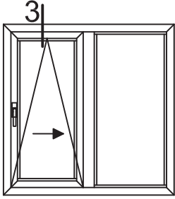
Tilt&Slide Parallel Lifting Sliding System Detail Paralel Devirmeli Sürme Sistem Detayı
