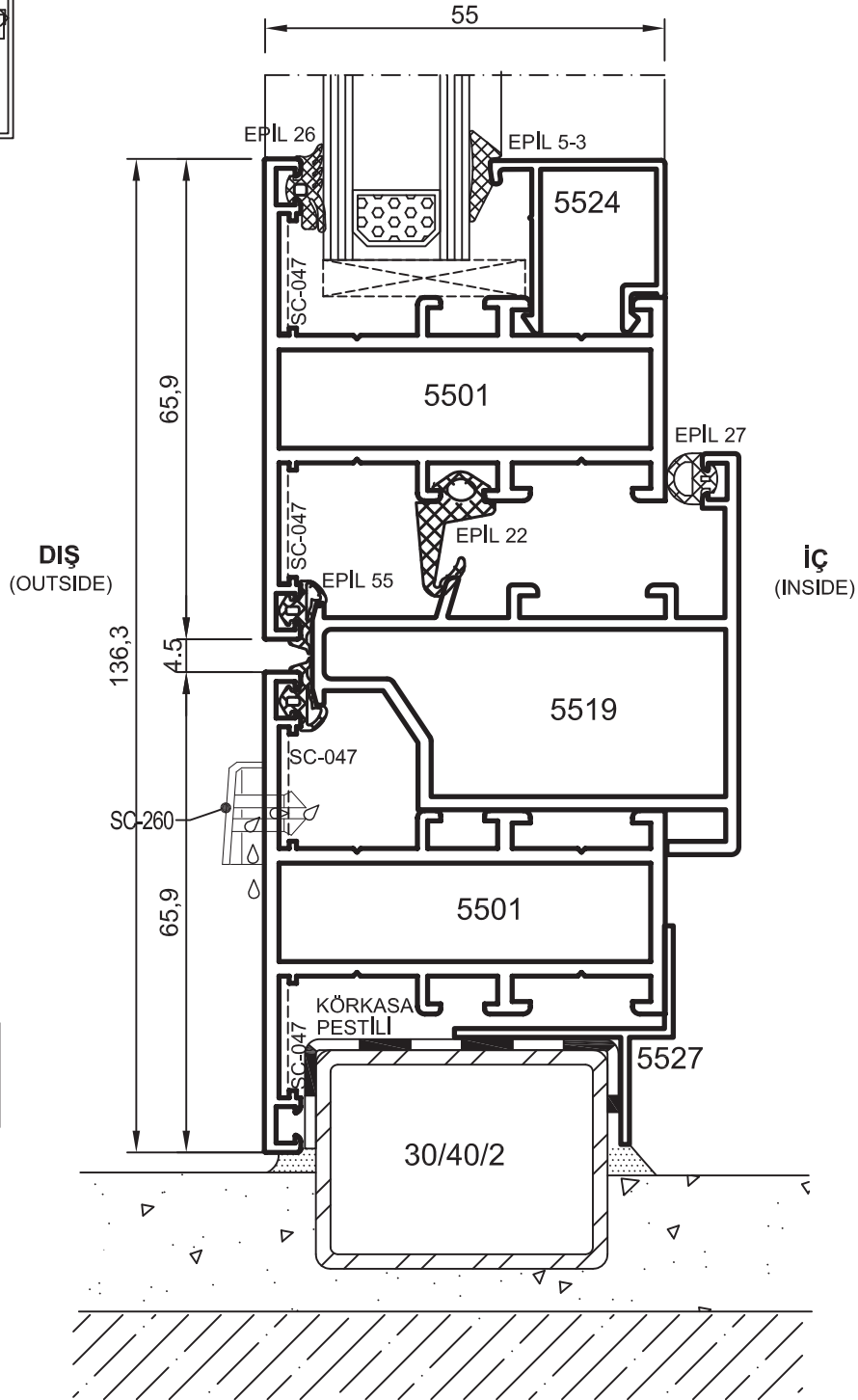
Pivot Window System Detail Pivot Pencere Sistem Detayı
